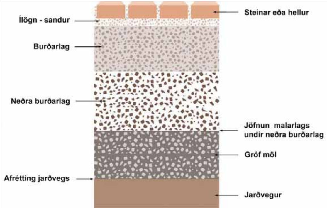
Erlend útlistun á uppbyggingu gangstéttar. Því vandaðri sem undirbyggingin er, þeim mun betur endist stéttin.
